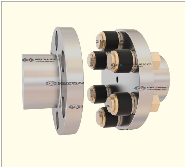
KFF Type
